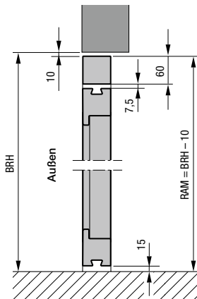
Vertikalschnitt
