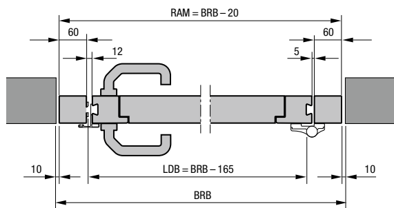
Horizontalschnitt
