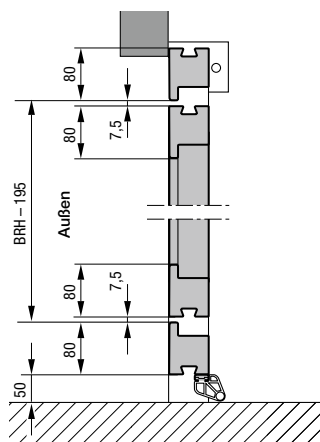
Vertikalschnitt
