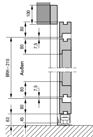
Vertikalschnitt
