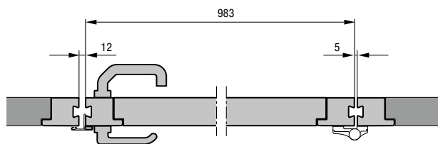
Horizontalschnitt
