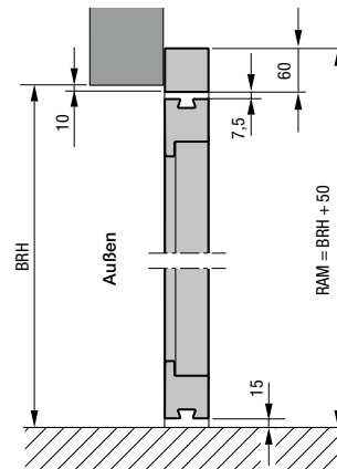
Vertikalschnitt
