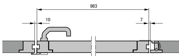
Horizontalschnitt
