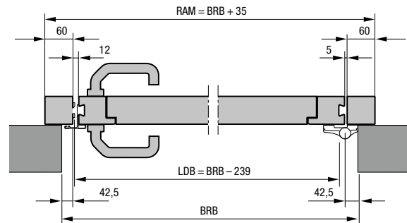
Horizontalschnitt
